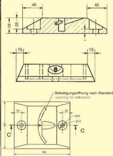
Detailzeichnung detail drawing
